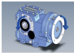
SENSO ORARIO RIFERITO ALL'ASSE VELOCE
