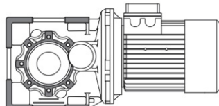
D FISSAGGIO PIEDE / ALBERO PIENO D
