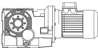
SL FISSAGGIO FLANGIA / ALBERO CALETTATORE L
