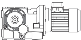
SS FISSAGGIO FLANGIA / ALBERO PIENO S
