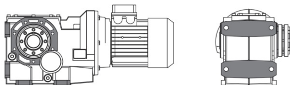
UL FISSAGGIO PIEDE-FLANGIA / ALBERO CALETTATORE L
