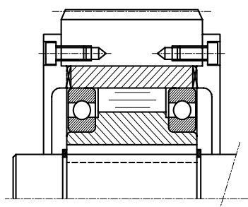
Esempio di montaggio Mounting example Exemple de montage
