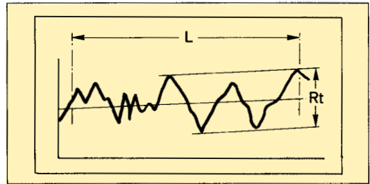
Fig. 20 - Misurazione della rugosità R_t .
