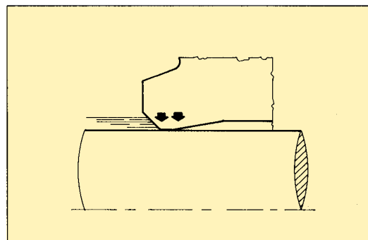
Fig. 11 - Carico radiale ottimale
