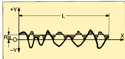
Fig. 21 - Misurazione della rugosità Ra.
