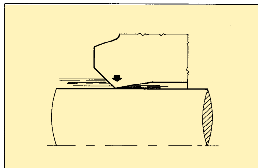
Fig. 9 - Carico radiale insufficiente
